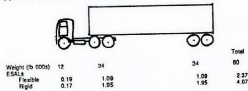
(d) Five-Axle Double (2-S1-2)
